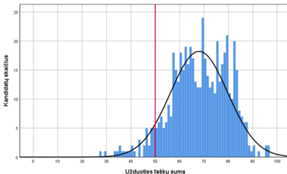
19 diagrama. Suvirintojo modulinės profesinio mokymo programos teorinės dalies (žinių) kompetencijų vertinimą laikusių asmenų surinktų taškų histograma.
